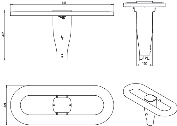
Dimensions / Mitat: GALAXY S4
