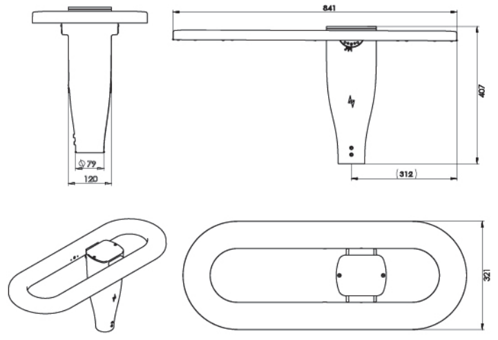
Dimensions / Mitat: GALAXY A4
