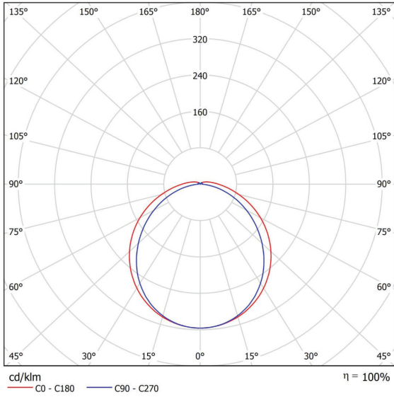
FL-HELIOS -valaisimien valonjakokäyrä ~112°
