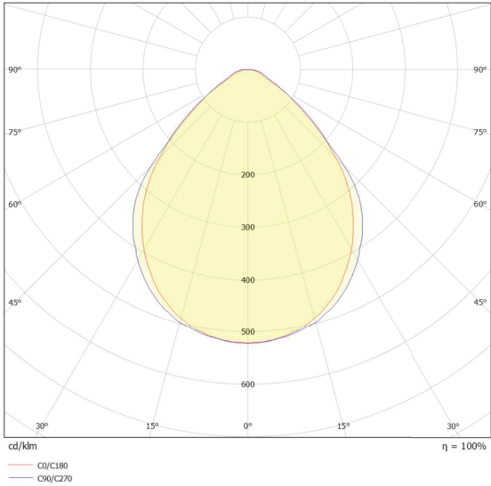
ALKES-S DPRZ-LT80
