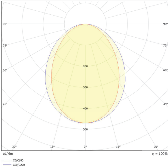
ALKES-S MPRZ-LT92
